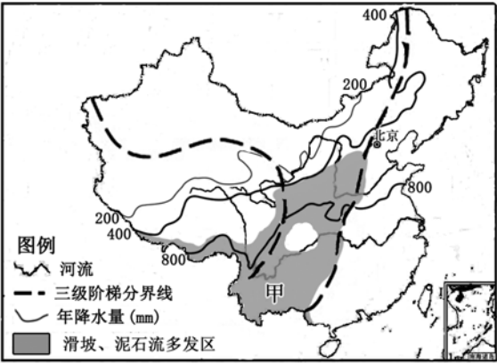
图 17 中国滑坡、泥石流多发区的分布图
